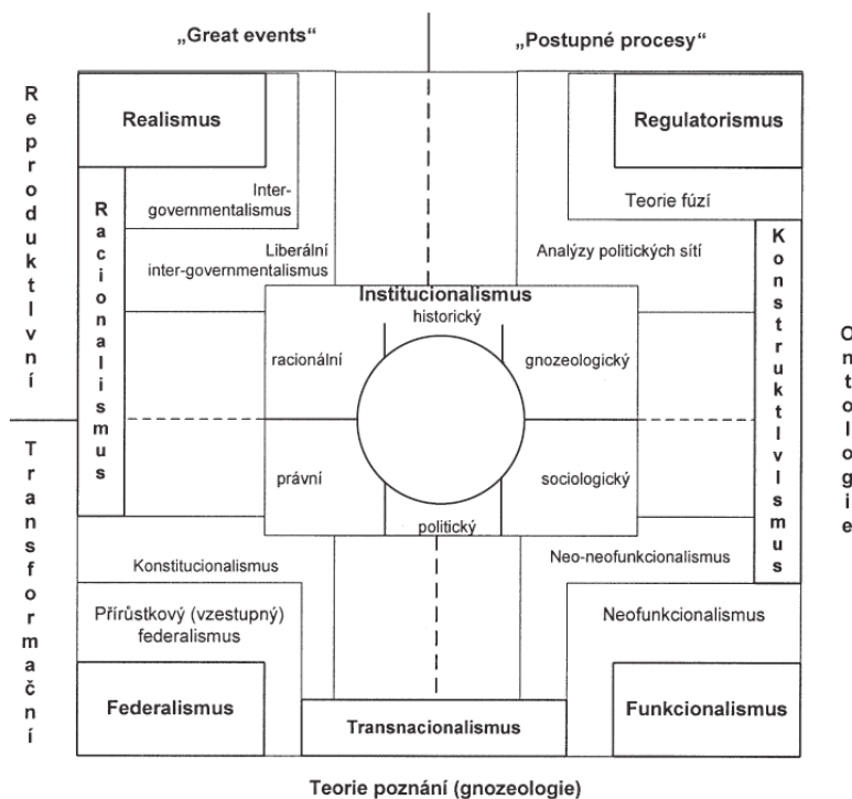
Obrázek 28: Teorie integrace
