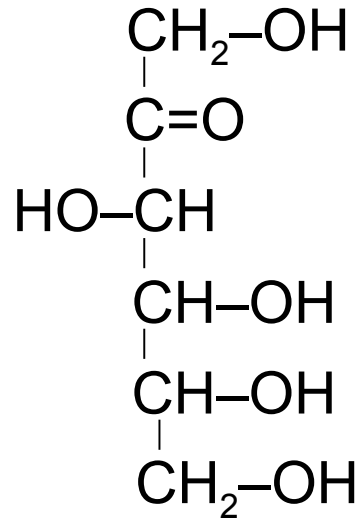
D-Fructose
