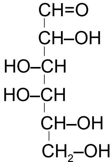
D-Galactose
