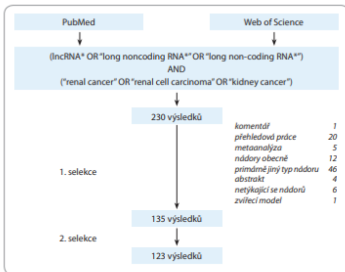
Obr. 1. Diagram vyhledávání.
