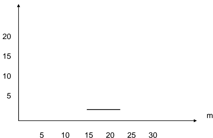
Graf výrobní izokvanty
