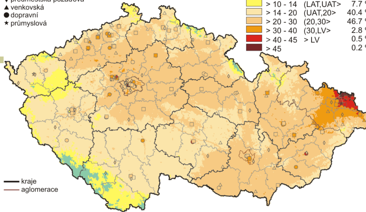
Pole roční průměrné koncentrace \text{PM}_{10} v roce 2007
