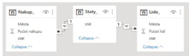
Tabulka Lide, Sloupec: Stat, Filtr: ČR
