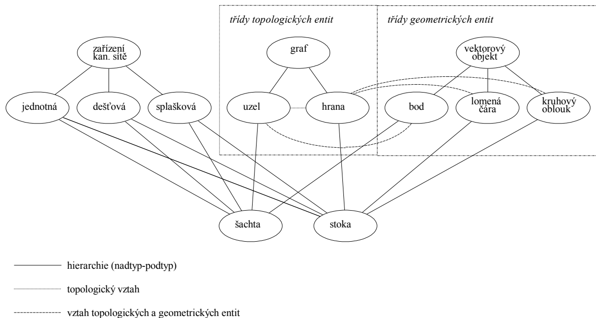
Obr. 24 - Příklad struktury jednoduchého datového modelu GIS
