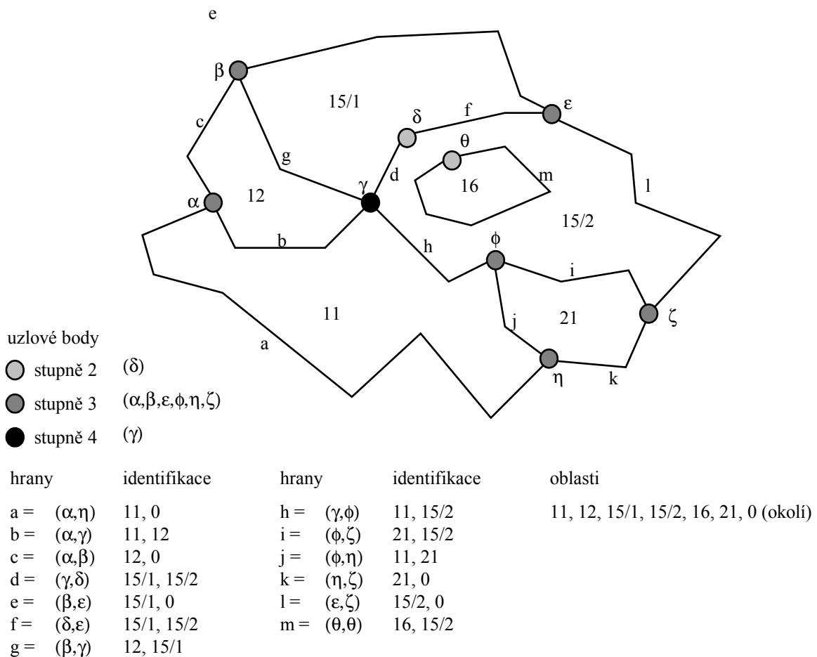
Obr. 26 - Příklad diagrafu rovinného areálového grafu
