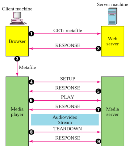
Obrázek: Příklad streamování uloženého videa s využitím protokolu RTSP.
