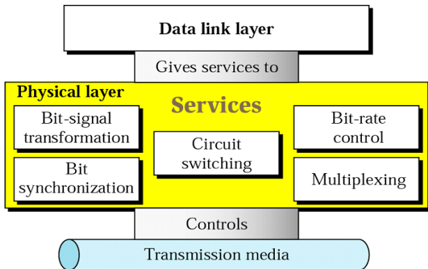
Obrázek: Ilustrace služeb fyzické vrstvy.
