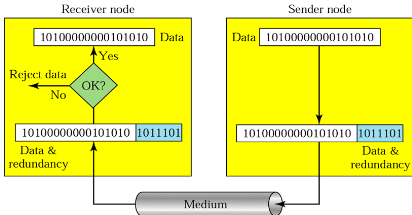
Obrázek: Proces detekce chyb – vysílač přidává k bloku bitů dat bity kódu pro detekci chyb (y).
