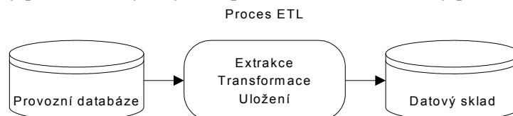
Obr.č.5 Obecné schéma datových skladů
