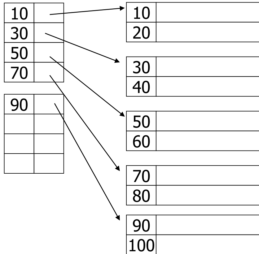
Index-sekvenční soubor
