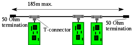
10Base2 Ethernet – schéma zapojení Zdroj: http://www.linuxfocus.org/
