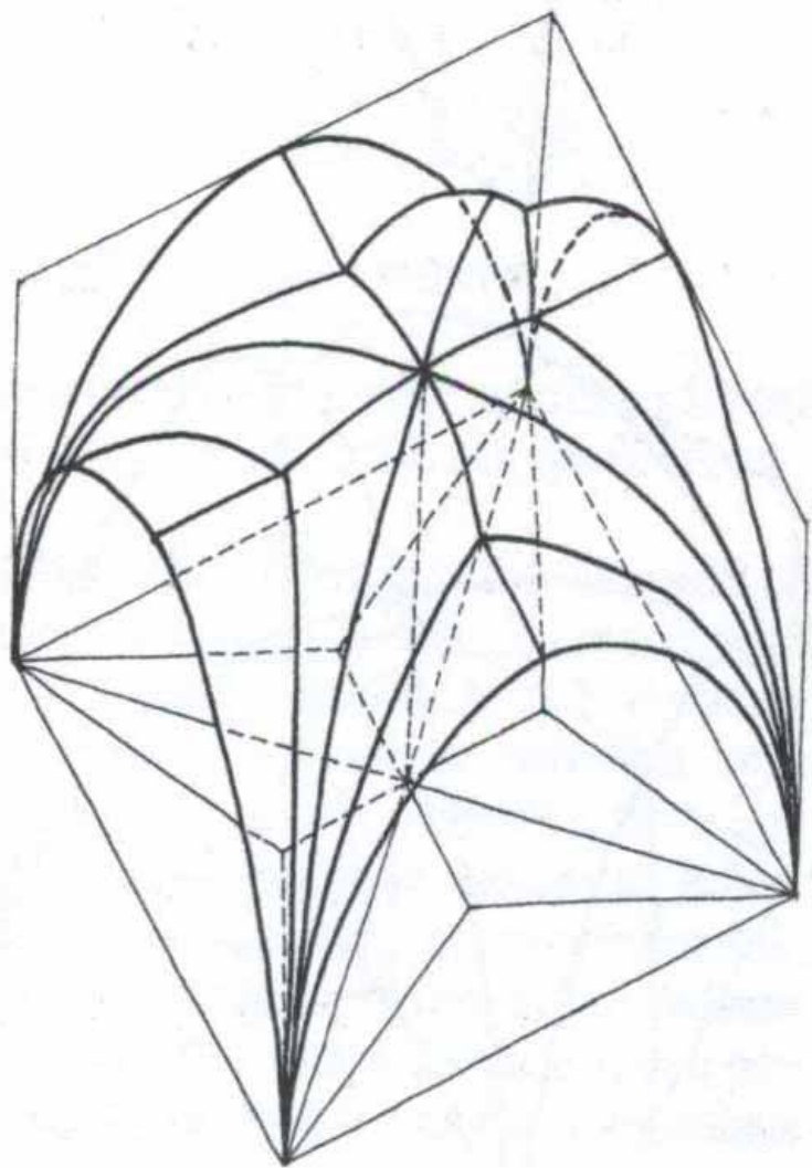
hvězdicová
