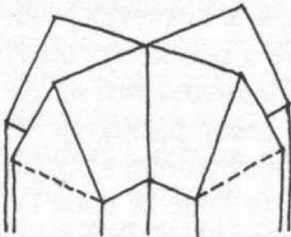
střecha křížová
