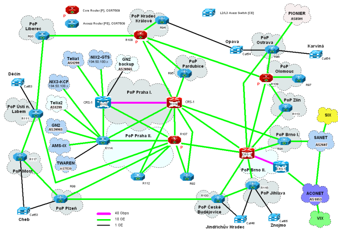
Figure: Logická topologie IP/MPLS vrstvy sítě CESNET2.
