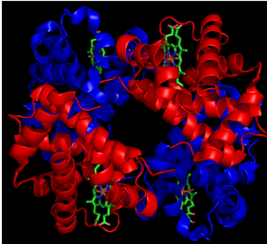
Struktura hemoglobinu: Proteiny 2x \alpha (červená) a 2x \beta (modrá) a hemové skupiny (zelená) (zdroj: wikipedia)
