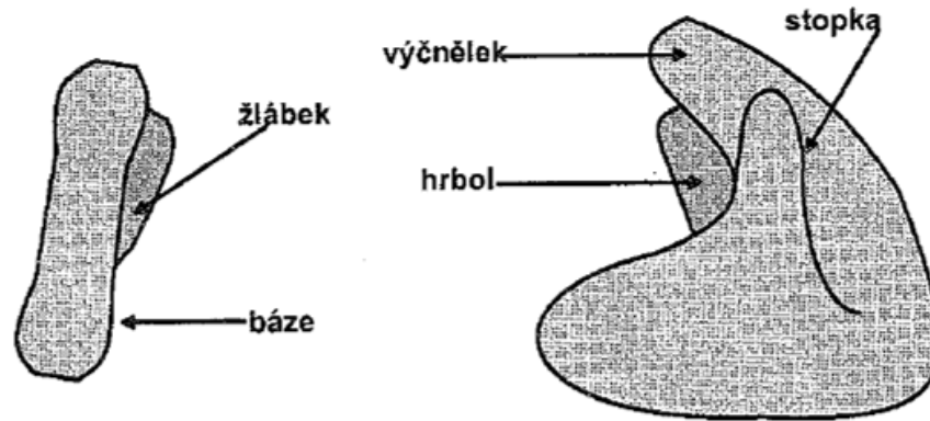
Podjednotka 30S
