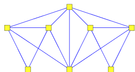
OBRÁZEK 1. Graf G_1
