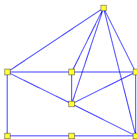
OBRÁZEK 2. Graf G_2
