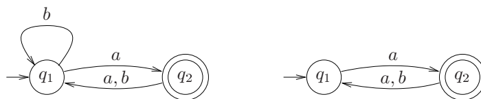
Obrázek 1.2: Automaty \mathcal{A} (vlevo) a \mathcal{B} (vpravo)
