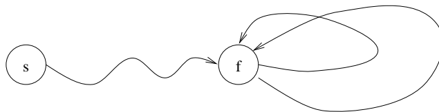
Obrázek 1.1: typický úspěšný běh Büchiho automatu, s \in S_{in} , f \in F
