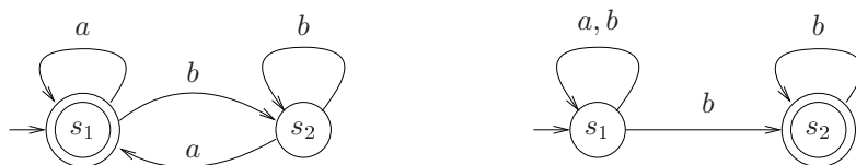
Obrázek 1.3: Automaty \mathcal{A}_1 (vlevo) a \mathcal{A}_2 (vpravo)
