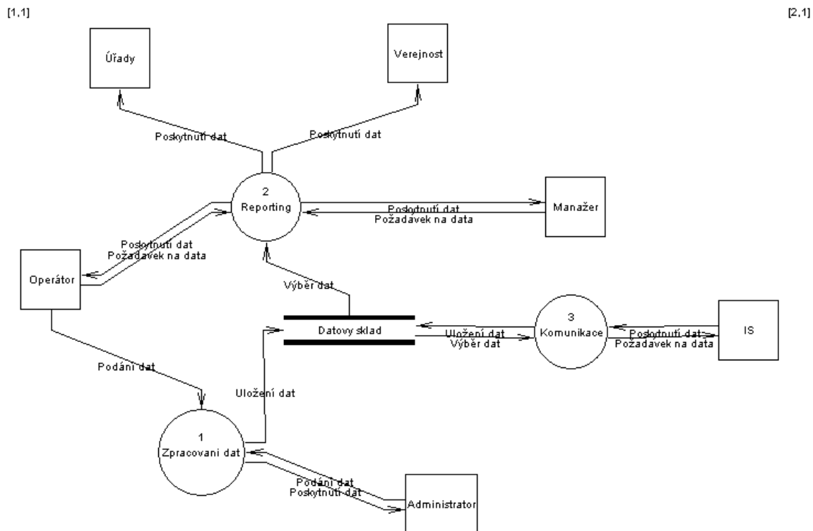
Obrázek č. 2: Diagram datových toků 1.úrovně
