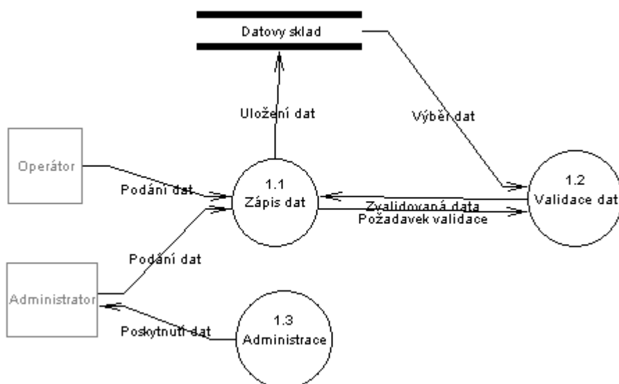
Obrázek č. 3: Diagram datových toků v procesu zpracování dat
