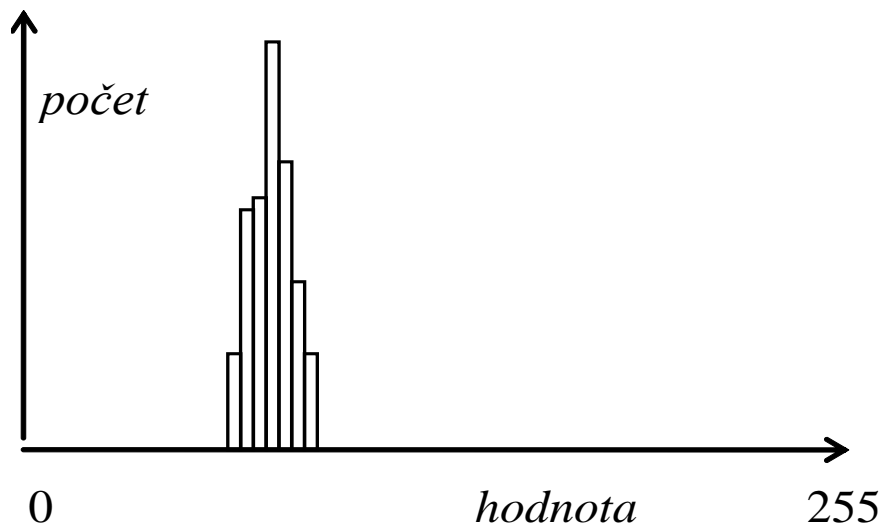
Obr. 18 - Histogram obrazu
