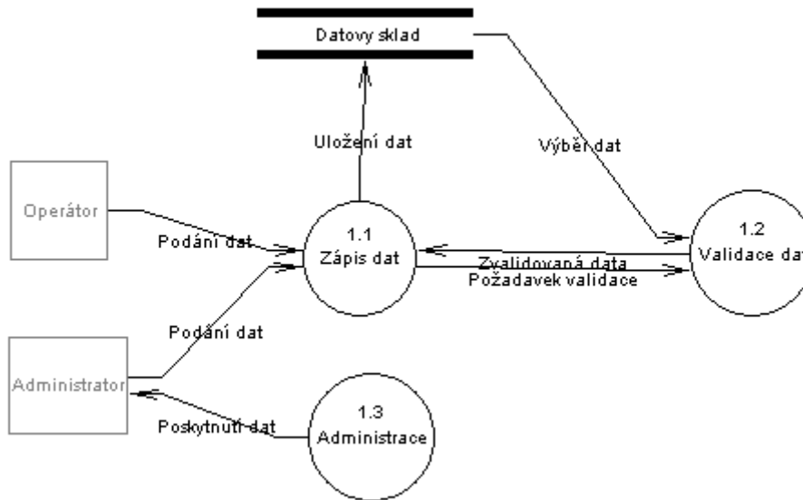
Obrázek č. 3: Diagram datových toků v procesu zpracování dat
