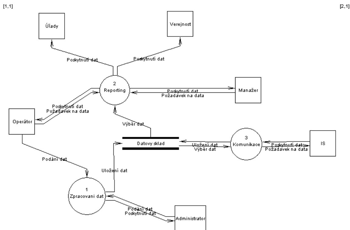
Obrázek č. 2: Diagram datových toků 1.úrovně
