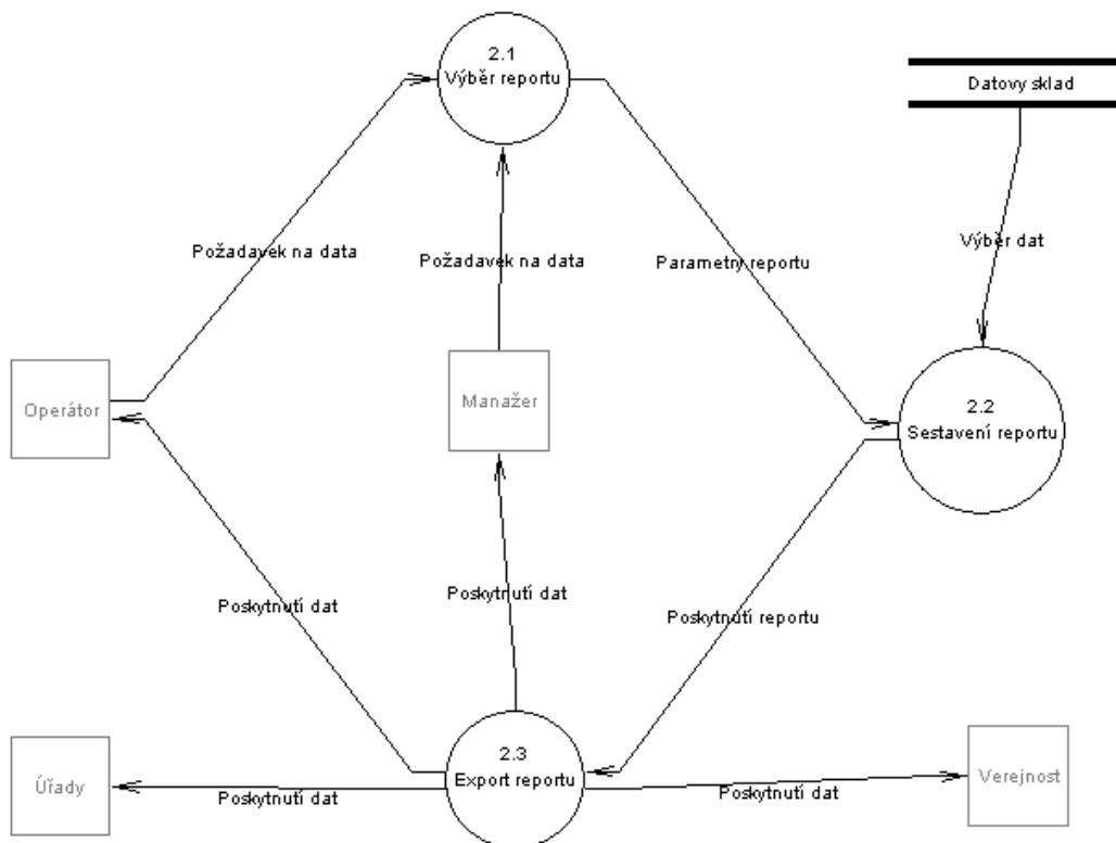
Obrázek č. 4: Diagram datových toků v procesu reporting
