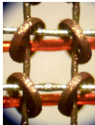
Detail čtyř buněk paměti (adresové vodiče a červený čtecí vodič) Zdroj: http://root.cz
