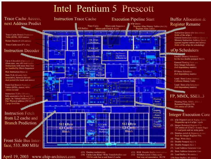
Jádro Prescott (90 nm)
