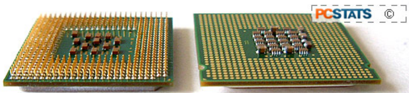
PGA vs. LGA – Zdroj: http://pcstats.com
