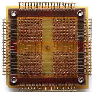
Feritová paměť o kapacitě 32×32 b Zdroj: http://en.wikipedia.org
