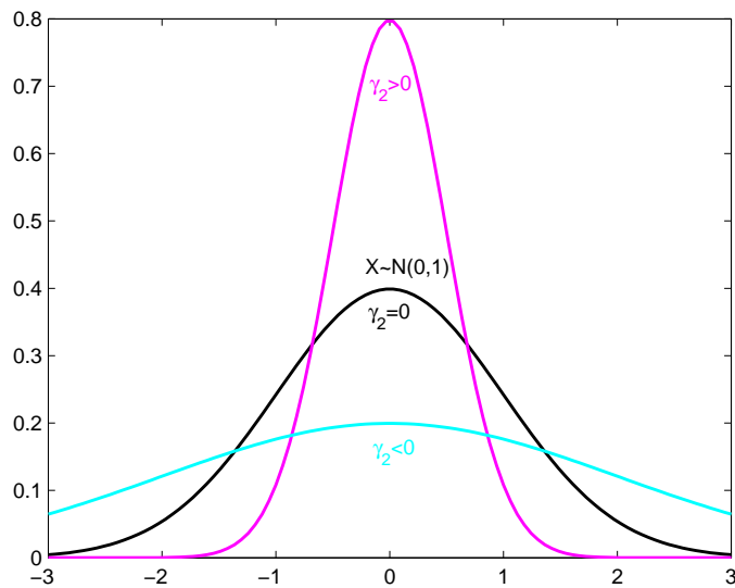
OBRÁZEK 3. Koeficient špičatosti
