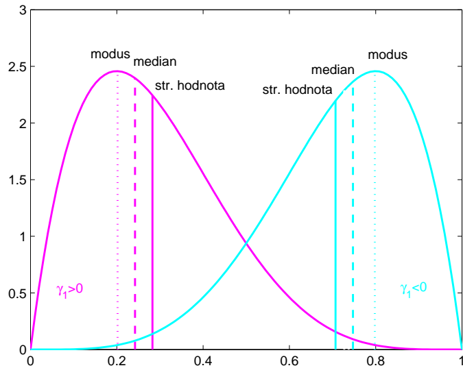
OBRÁZEK 2. Koeficient šikmosti
