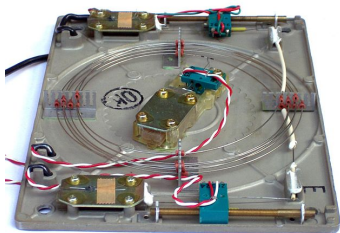
Magnetorestriktivní cívka (60. léta) Zdroj: http://en.wikipedia.org
