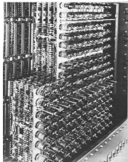
Větší blok operační paměti sestavený z triod Zdroj: http://root.cz
