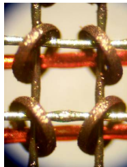
Detail čtyř buněk paměti (adresové vodiče a červený čtecí vodič)
