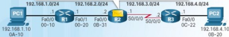
Layer 2 Data Link Frame
