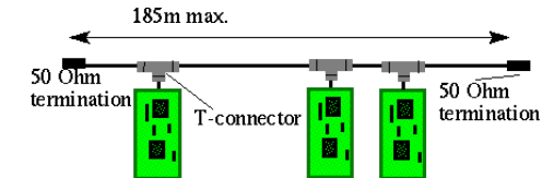
10Base2 Ethernet – schéma zapojení Zdroj: http://www.linuxfocus.org/
