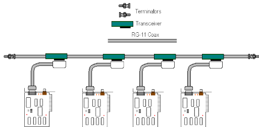
10Base5 Ethernet – schéma zapojení Zdroj: http://physinfo.ulb.ac.be
