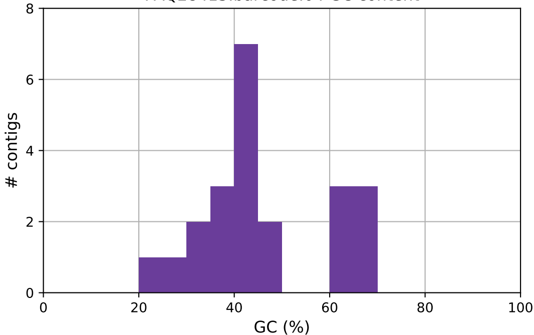
FAQ28413.barcode.04 GC content
