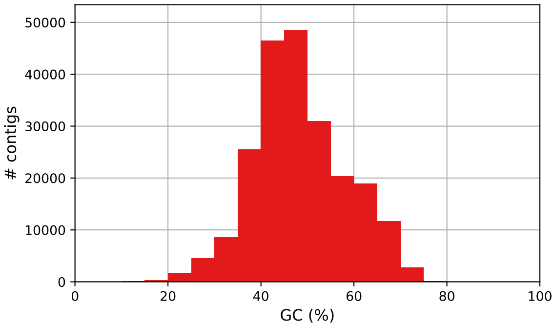
FAQ28413.barcode.01 GC content
