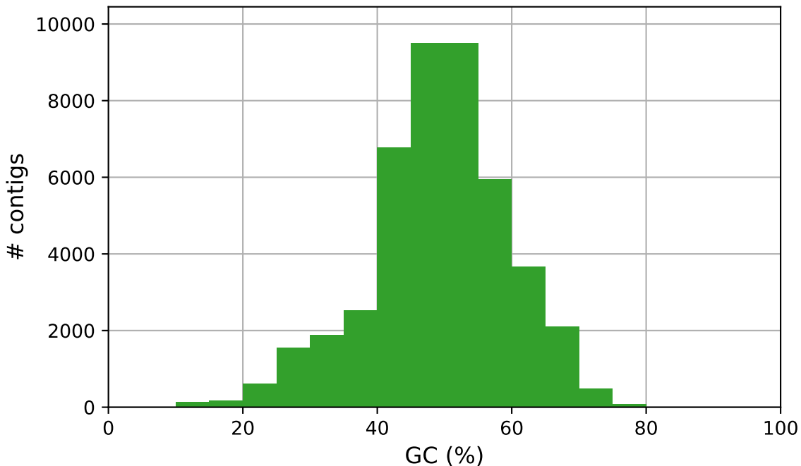
FAQ28413.barcode.03 GC content
