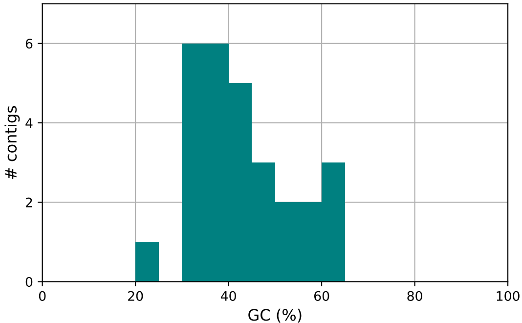
FAQ28413.barcode.12 GC content
