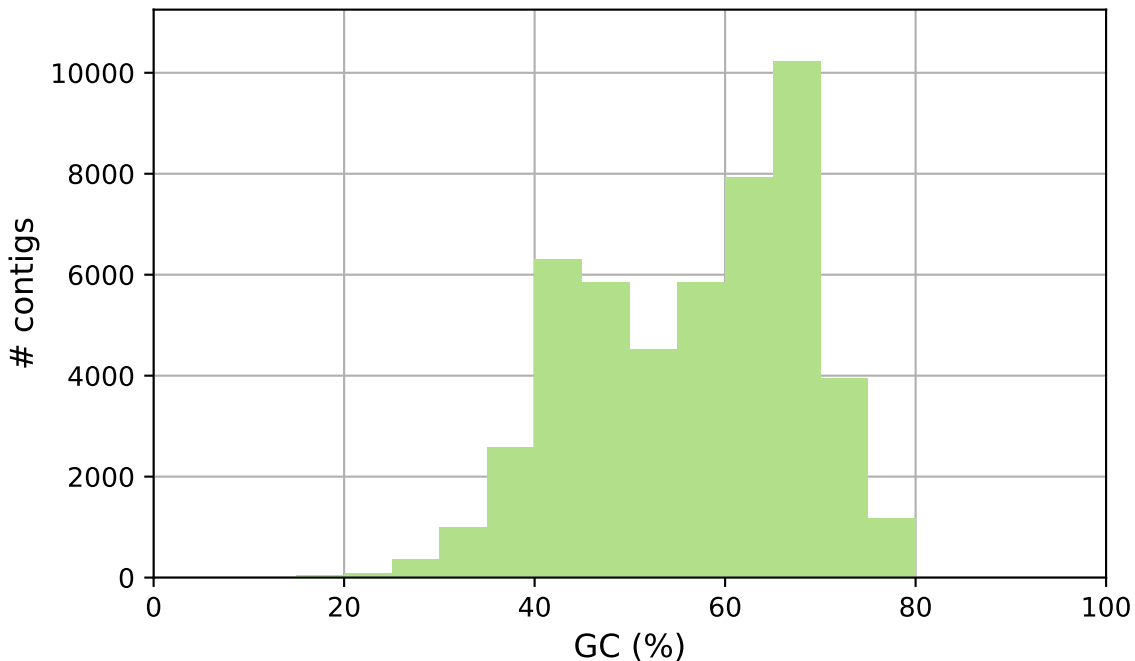
FAQ28413.barcode.08 GC content
