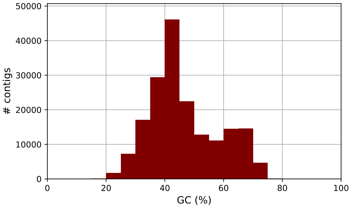
FAQ28413.barcode.06 GC content
