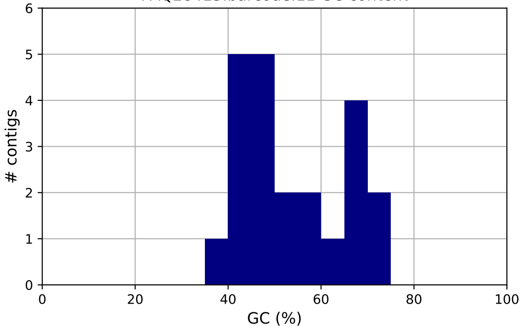
FAQ28413.barcode.11 GC content
