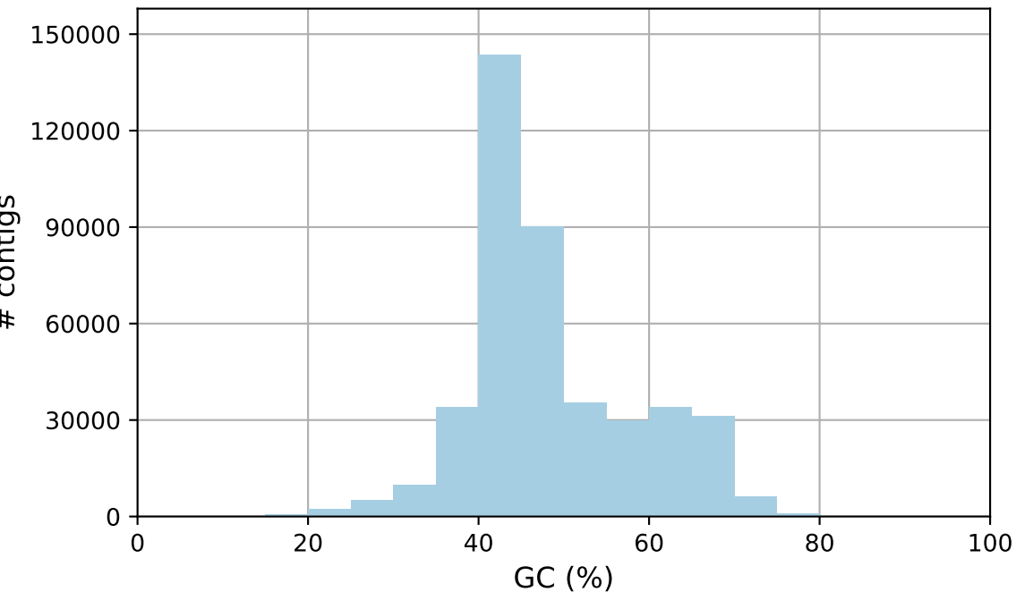
FAQ28413.barcode.07 GC content
