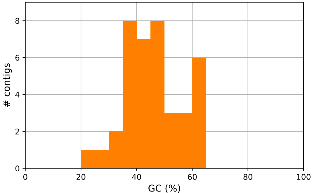
FAQ28413.barcode.05 GC content
