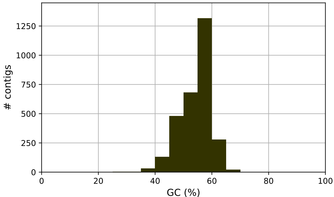
FAQ28413.barcode.09 GC content
