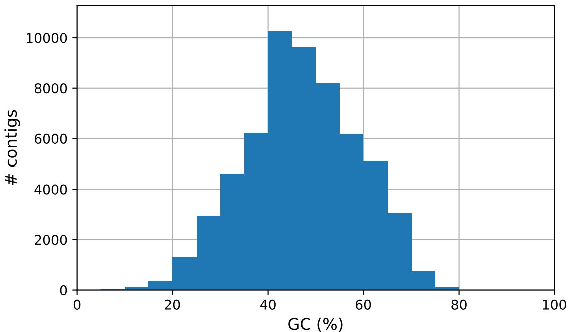
FAQ28413.barcode.02 GC content
