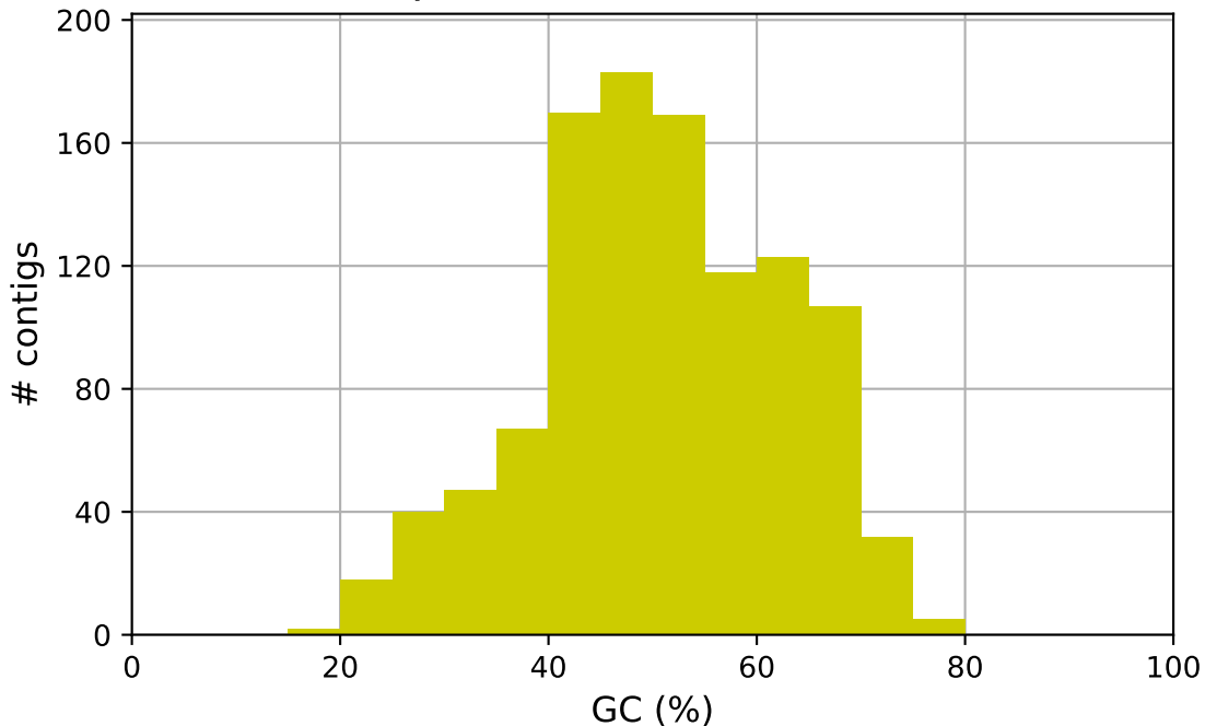
FAQ28413.barcode.10 GC content
