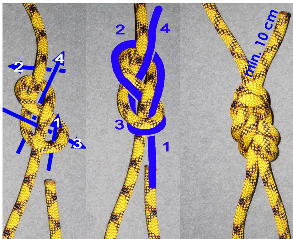
obr. 4 – Vyvázání dvojitěho osmičkového uzlu kopírováním
