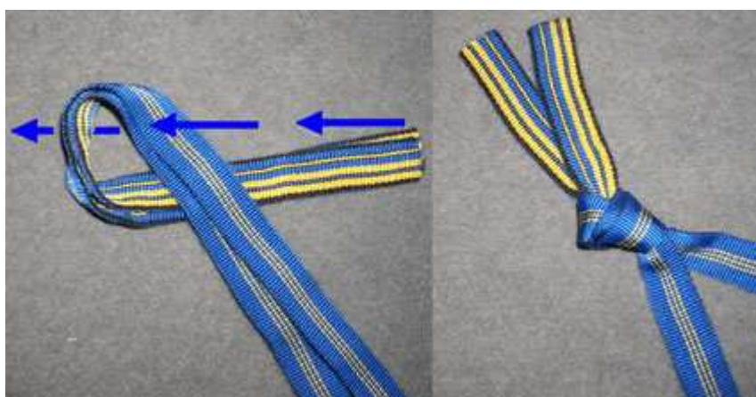
obr. 23 – Vűdcovský uzel stejnosměrný
