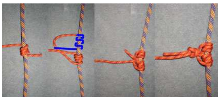
obr. 34 – Trojitý Prusíkův uzel vyvazaný z jednoho pramene smyčky
