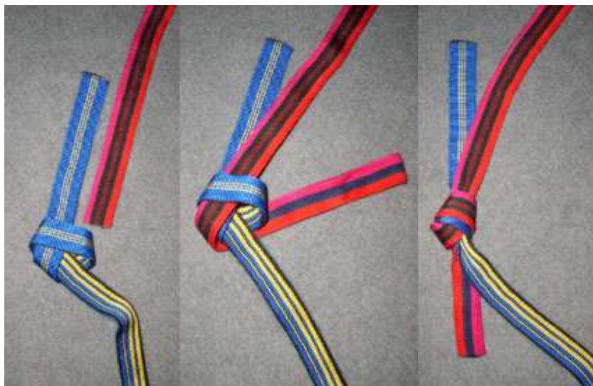
obr. 22 – Vűdcovský uzel profisměrný (skotský)
