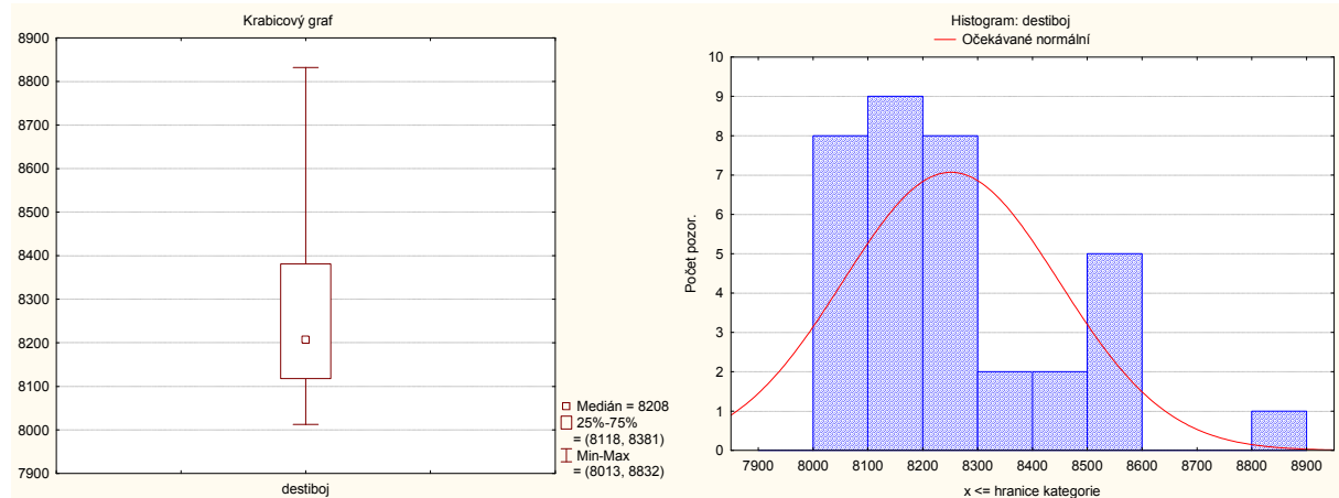
Obr. 47. Krabicový graf
