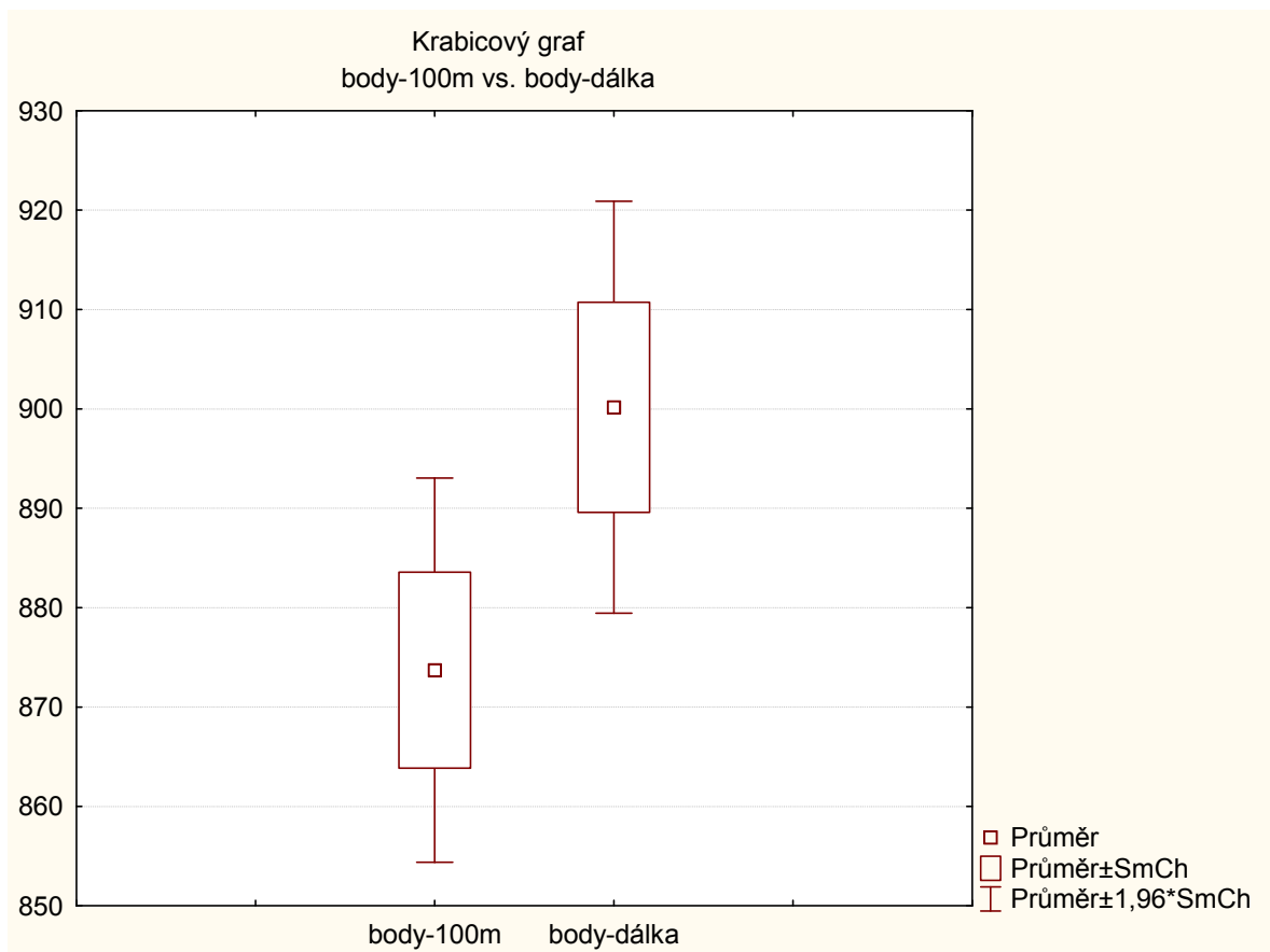
Obr. 50. Krabicový graf
