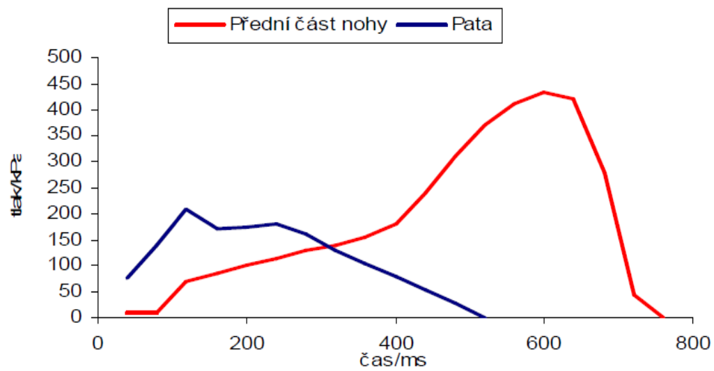
Obr. 18: Graf závislosti maximálních hodnot tlaku na čase – levá noha
