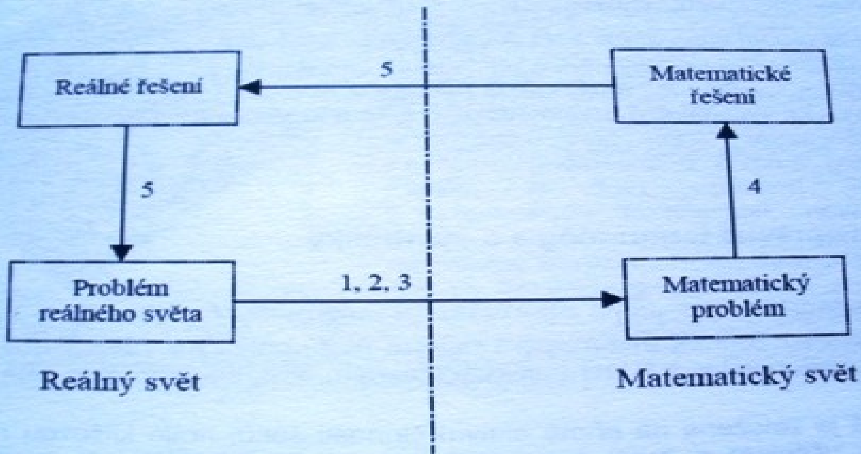
Obr. 1: Cyklus matematizace [12]
