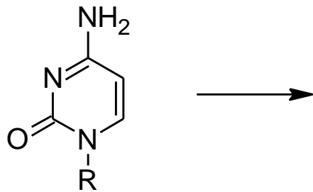
cytosin
