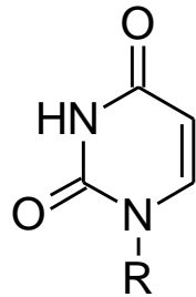
uracil
