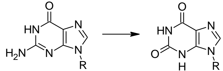
guanin
