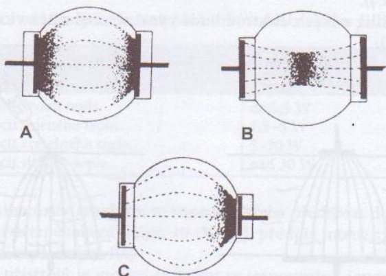
Obr. 8.6 Vliv velikosti elektrod a jejich vzdálenosti na hloubku účinku KVD: A – stejně velké elektrody, těsně u povrchu, B – stejně velké elektrody, obě oddáleny, C – nesterjně velké elektrody, nesterjně oddáleny
