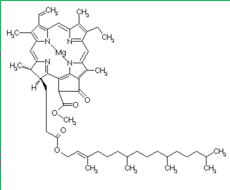
chlorofyl a
