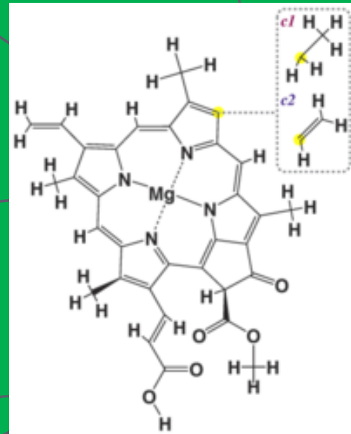
chlorofyl c
