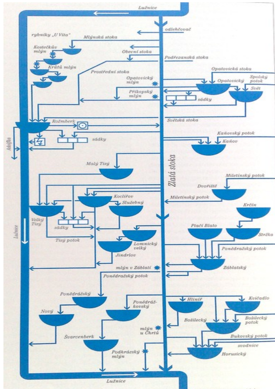
Vodohospodářské schéma napájení rybníků Zlatou stokou. Rybníky jsou znázorněny jako nádoby, jimiž voda kaskádovitě protéká. Proto je i směr toků zobrazen shora dolů. Ve skutečnosti tečou Zlatá stoka i Lužnice k severozápadu. (Kresba A. Pokorné, podle A. Kalného ml.)
