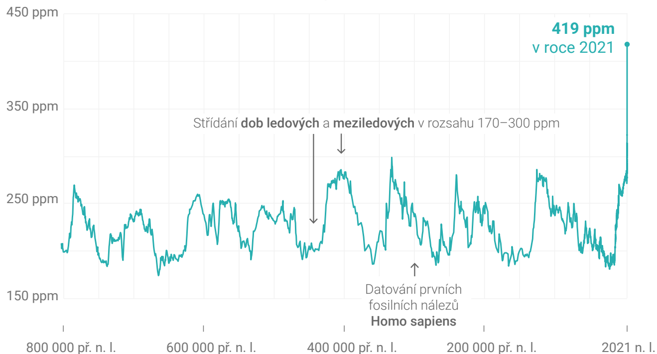
Koncentrace CO 2 za posledních 800 000 let
