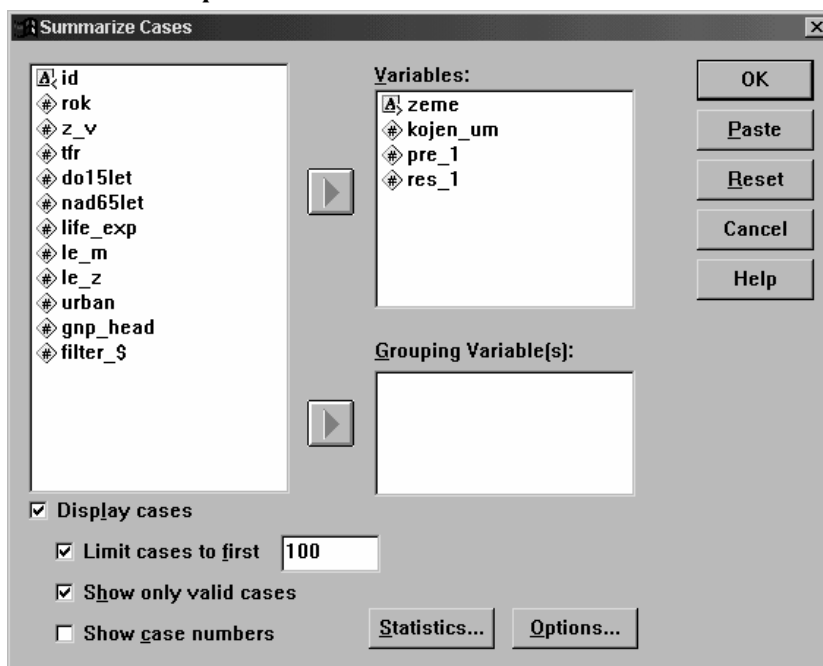
Obr. 10.7: Dialogové okno pro zobrazení hodnot nezávisle a závisle proměnné, rekonstruovaných hodnot závisle proměnné a reziduí
