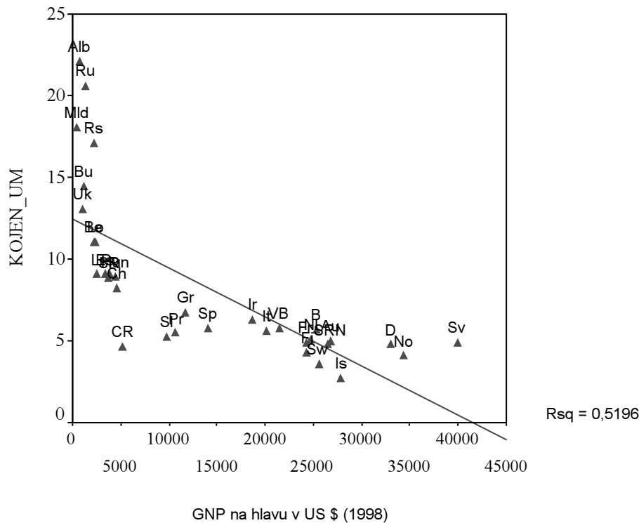
Obr. 11. 3: Regresní přímka popisující vztah mezi urbanizací a populačním stárnutím
