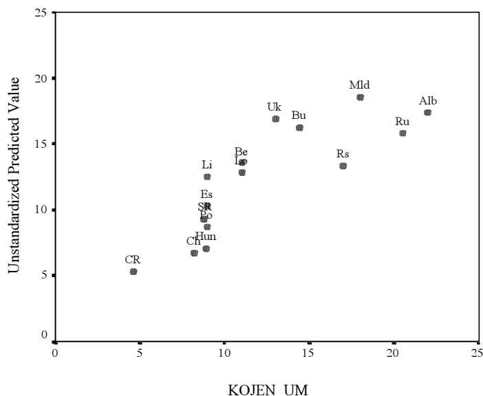
Obr. 11. 8: Graf predikovaných hodnot (pre_1) oproti hodnotám závisle proměnné
