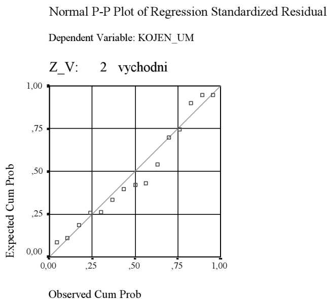
Obr. 11. 10: Graf pravděpodobnosti normality rozložení reziduí
