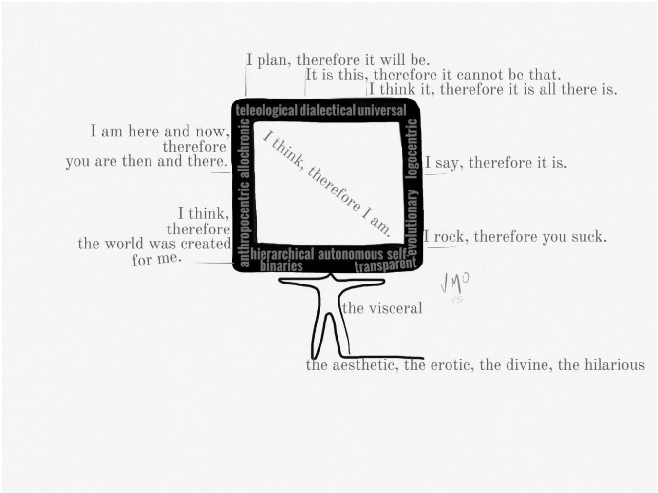
Obr. 1 Karteziánské já
