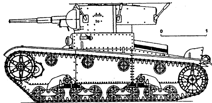
Bokorys tanku T-26 vzor 1933
