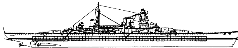
Těžký křižník typu „Kronštadt“ (projekt 69)
