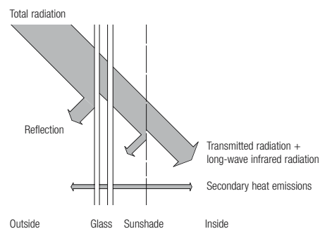
Fig. 75: Internal sunshade
