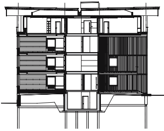
Fig. 263: Section A-A
