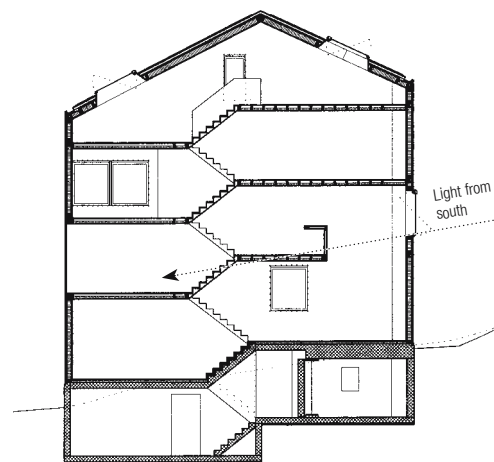
Fig. 294: Longitudinal section
