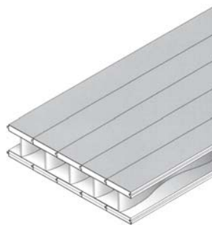
Fig. 34: Wellsteg hollow element
