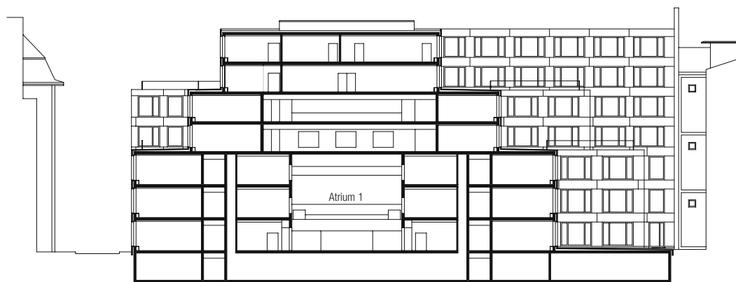
Fig. 189: Longitudinal section, 1:600
