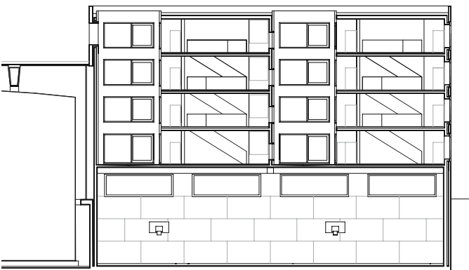
Fig. 159: Longitudinal section, 1:500
