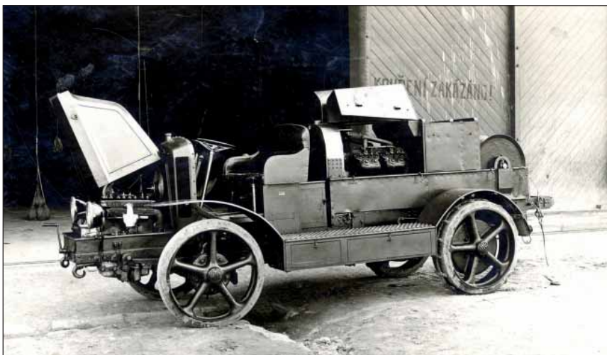
Speciální navíjecí vůz značky Latil určený k manipulaci s pozorovacími balóny. Byl zařazen ve stavu balónové roty 1.
