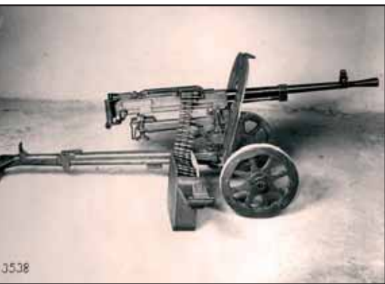
Těžký kulomet Gorjunov vz. 43 S
