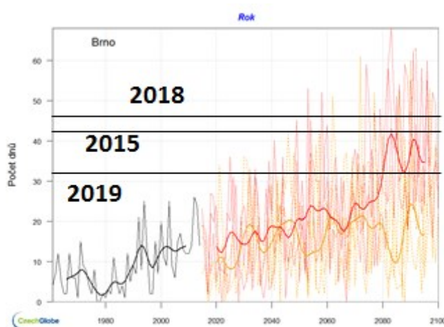
Obr. 2a Vývoj počtu dnů s tropickou teplotou (nad 30°C) pro 2 scénáře: Červená křivka je pro situaci, kdy se nepodaří snížit emise, žlutá křivka pro scénář s podstatným snížením emisí. Vyobrazení ensamblu souborů variant scénářů s výrazným rozptylem. Zdroj: Czech Globe, ČHMÚ a Mendelova univerzita.
