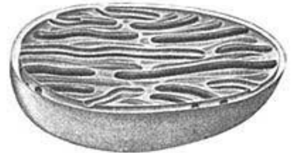
tubulózní kristy
