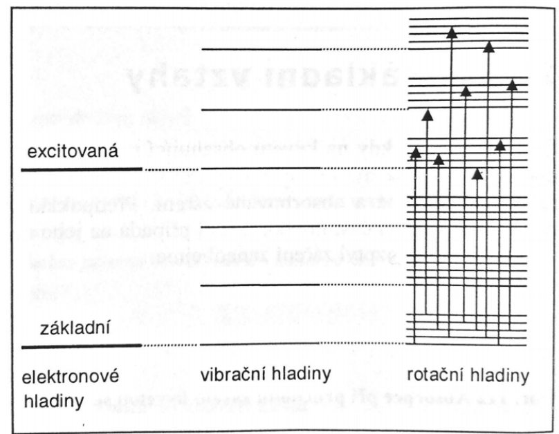
schéma přechodů elektronu při absorpci UV/VIS
