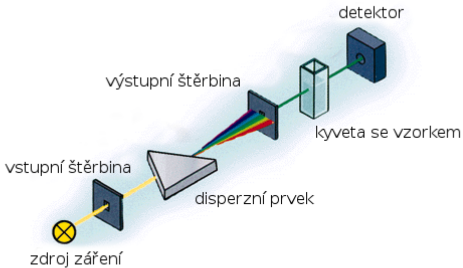
základní schéma spektrofotometru
